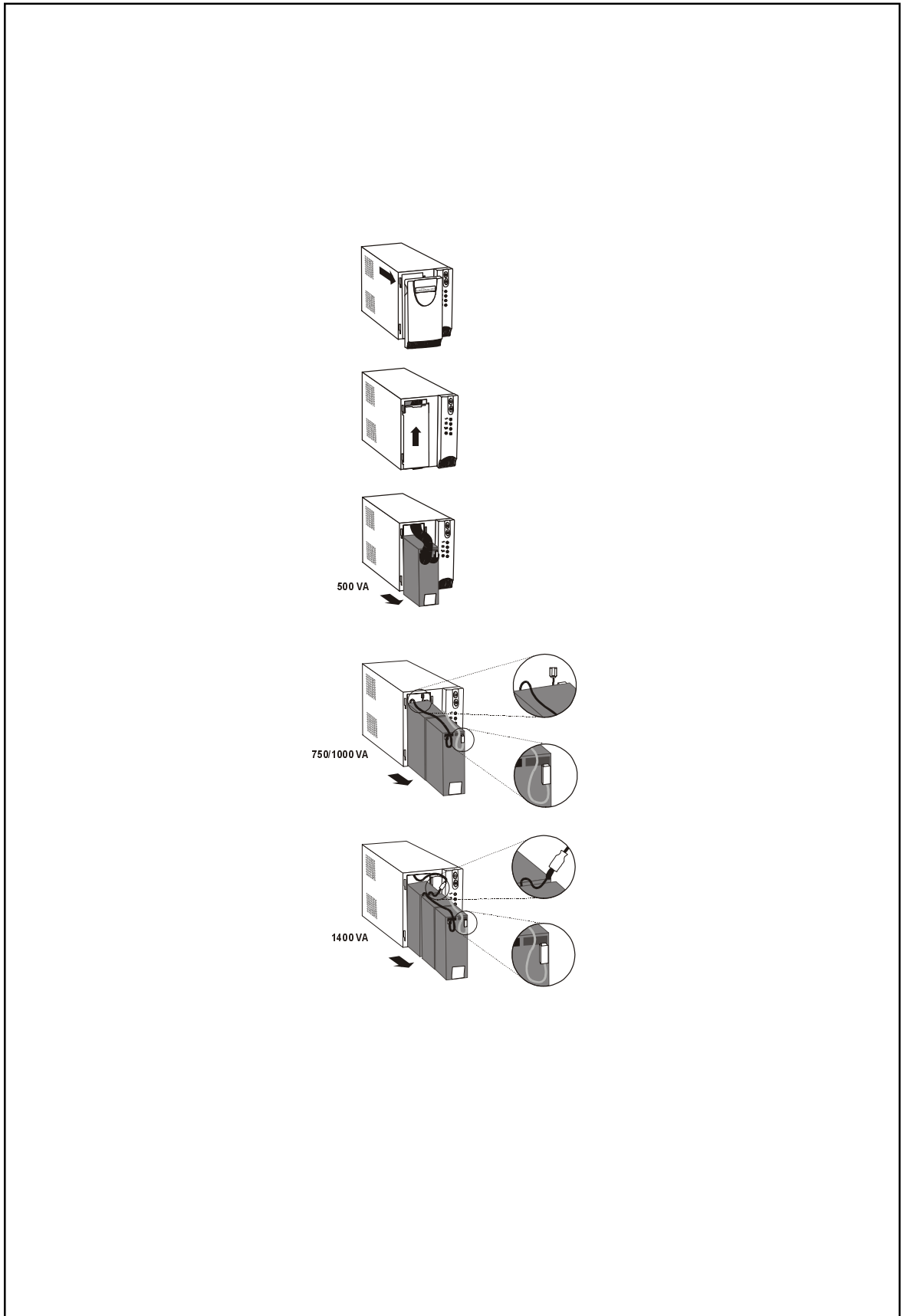
Fig. 8. Remplacement des batteries.
