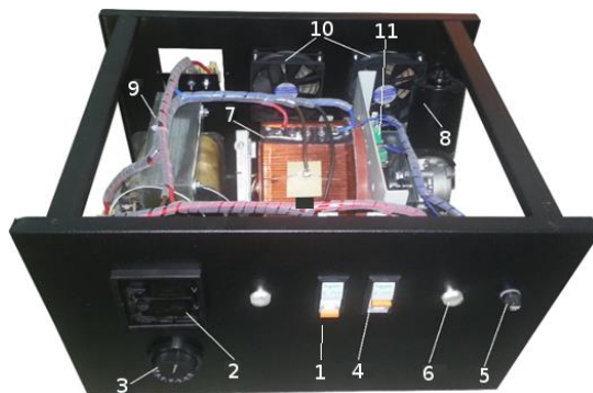
Régulateur monophasé de 1 à 50KVA
