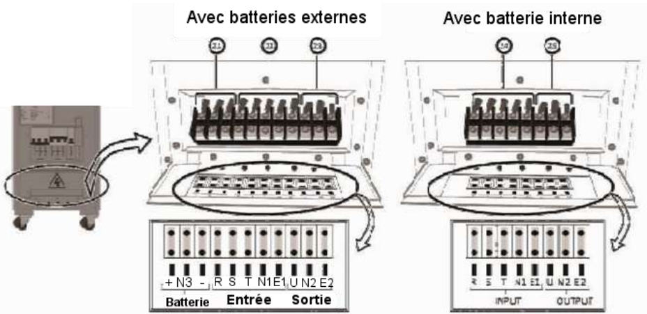
Figure-4 vue arrière et connexion de l'onduleur
